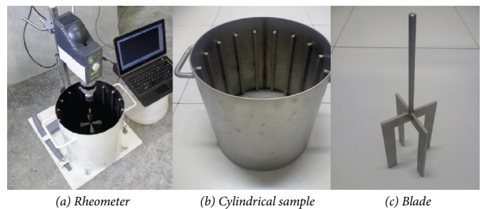
Fig. 6 The configuration of the rheometer used and its constituents [21] 6. ábra Az alkalmazott reométer mérési összeállítása és alkotóelemei [21]
