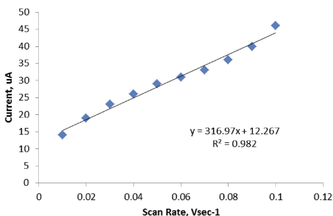
Fig. 11 Plot the reduction current peak of K_4[Fe(CN)_6] at different scan rates on working electrode of polyacrylonitrile self-modified with CNT 11. ábra K_4[Fe(CN)_6] redukciós áramcsúcsa különböző mintavételi sebesség mellett CNT-vel módosított polimer elektródat használva
