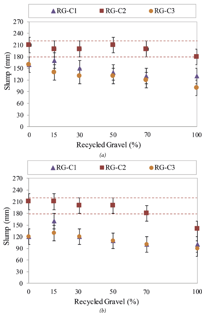
Fig. 2 Variation of slump with percentage of substitution in RG: (a) T30; (b) T90 2. ábra A roskadás változékonysága az újrahasznosított durva adalékanyag (RG) mennyiségének függvényeként: (a) T30; (b) T90
