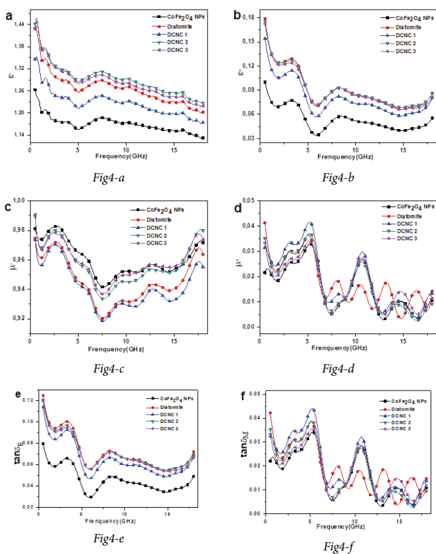
4. ábra A \text{CoFe}_2\text{O}_4 NP-k, a diatomit és a DCNC dielektromos tulajdonságai. DCNC 1 és DCNC 3 \text{CoFe}_2\text{O}_4 NP-k, a diatomit aránya 1:2, 1:5, illetve 1:10 között. Komplex permittivitás ( \epsilon' , a, b), komplex permeabilitás ( \mu' , c, d) és veszteségtangens ( \tan \delta_E , e, f). Az \epsilon' ( \epsilon' , a) valódi része, az \epsilon'' ( \epsilon'' , b) képzetes része. \mu' ( \mu' , c) valódi része, \mu'' ( \mu'' , d) képzetes része. Elektromos veszteségtangens ( \tan \delta_E , e), mágneses veszteségtangens ( \tan \delta_M , f)
