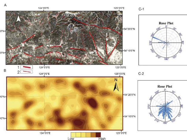
5. ábra A vizuális vonal-elemzés eredményei. A - LANDSAT 8 (7,4,2 sávok): 1 - 1. rangsor vonalak, 2 - 2. rangsor vonalak; B - a vonalak térbeli sűrűsége; C-1 - Rose plot az 1. rang; C-2 - Rose plot a 2. rang Fig. 5 Results of the visual lineament analysis. A - LANDSAT 8 (7,4,2 bands): 1 - 1 st rank lineaments, 2 - 2 nd rank lineaments; B - Spatial density of lineaments; C-1 - Rose plot for 1 st rank lineaments; C-2 - Rose plot for 2 nd rank lineaments
