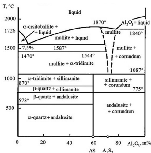
1. ábra SiO 2 -Al 2 O 3 rendszer normál körülmények között (átvéve L. Gömze A., 2001 [16] N M Bobkova 2007 [17])
