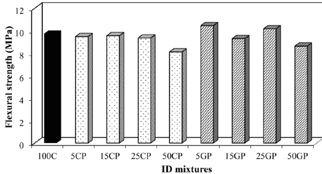
Fig. 9 Flexural strength for mortar mixtures with plain and blended cements at 56 days 9. ábra Hajlítási szilárdság habarcskeverékekhez sima és kevert cementekkel 56 napos korban
