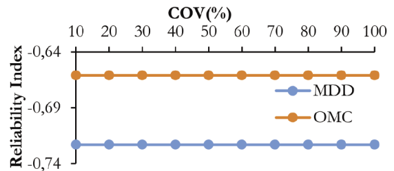
Fig. 8 Relationship between reliability index and COV for fine content 8. ábra A megbízhatósági index és a COV közötti összefüggés a finomrésztartalomhoz
