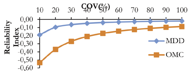
Fig. 9 Relationship between reliability index and COV for specific gravity 9. ábra A megbízhatósági index és a COV közötti összefüggés a fajtsúlyhoz
