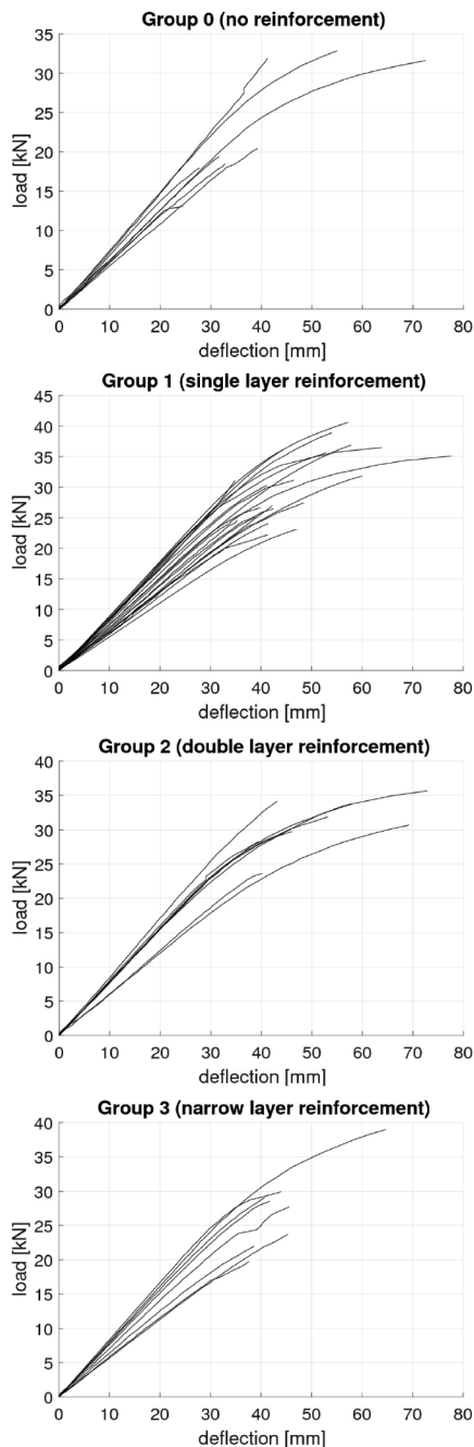
Fig. 3 Load-deflection curves for all specimen groups. 3. ábra Erő-lehajlás-görbék minden tesztszoportban.
