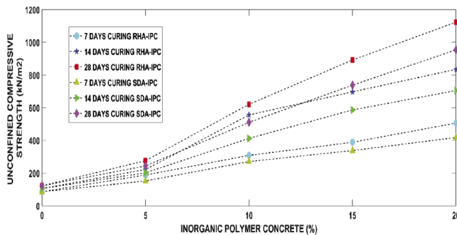
Fig. 5 UCS of natural and inorganic polymer cement modified black cotton soil 5. ábra Természetes és szervesetlen polimer cementtel módosított fekete pamut talaj UCS
