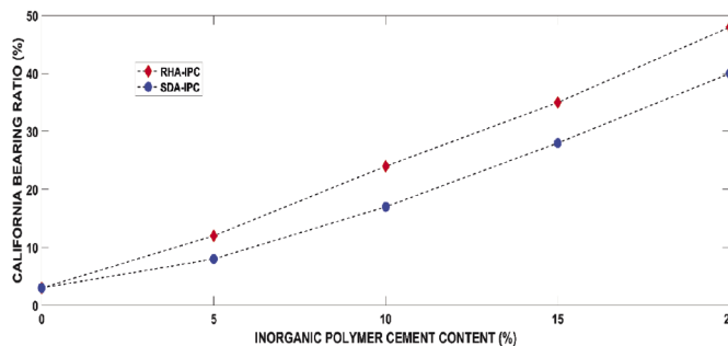
Fig. 6 CBR of natural and inorganic polymer cement modified black cotton soil 6. ábra Természetes és szervesetlen polimer cementtel módosított fekete pamut talaj CBR
