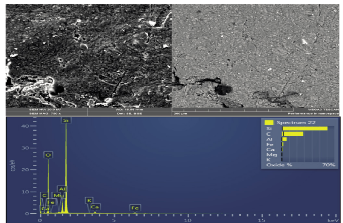
Fig. 8 SEM and EDS of 10% IPC-RHA treated BCS 8. ábra 10%-os IPC-RHA-val kezelt BCS SEM és EDS felvétele
