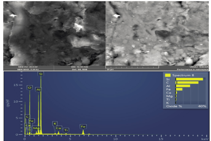
Fig. 7 SEM and EDS of natural BCS 7. ábra Természetes BCS SEM és EDS felvétele
