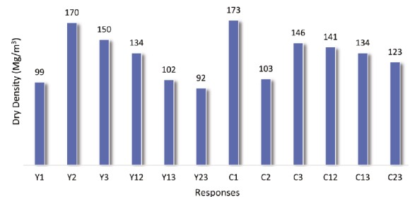
Fig. 5 Variations of Dry Density 5. ábra A száraz sűrűség változása
