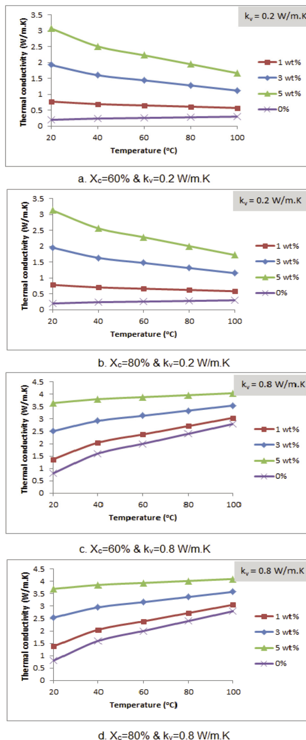
Fig. 1 Overall thermal conductivity of perovskite cell at different PEO concentrations 1. ábra Perovskit cella teljes hővezetési képessége különböző PEO koncentrációk mellett
