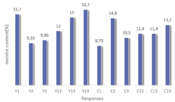
Fig. 4 Variations of Average Moisture Content 4. ábra Az átlagos nedvességtartalom változása
