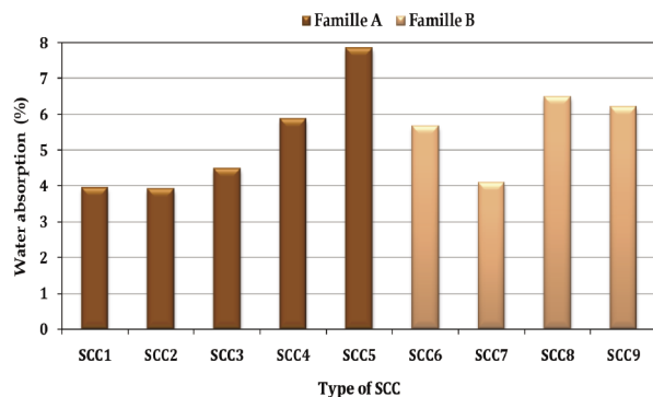
Fig. 6 Water absorption by immersion of SCC mixtures 6. ábra Az öntömörödő betonkeverékek (SCC) vízfelvetele vízbe merítéssel
