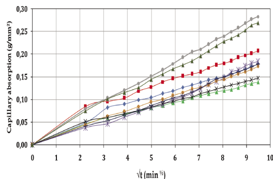
Fig. 7 Water absorption by capillarity of SCC mixtures 7. ábra Az öntömörödő betonkeverékek (SCC) kapilláris vízfelvetele
