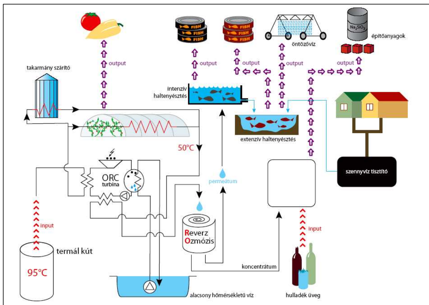
2. ábra: A geotermikus energia és a termálvíz többlépcsős komplex hasznosítása és a használt termálvíz környezetkímélő elhelyezése vizes élőhelyeken (Forrás: Salamon, 2007; Csürhész és mtsai, 2008)
