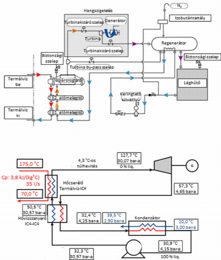
2. ábra: Az erőművi folyamat és az izobutánkör (IC4) nyomásai és hőmérsékletei
