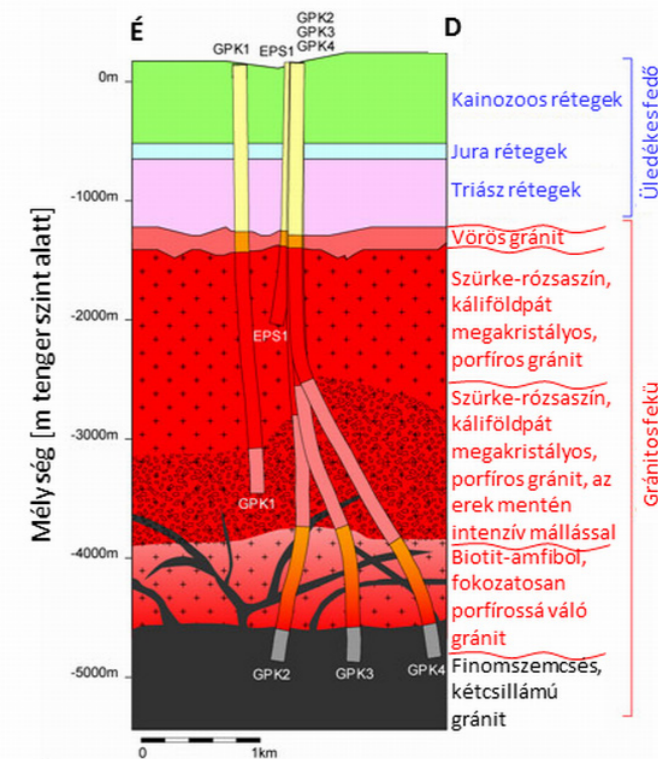
1. ábra: Soultz geológiája és a kutak elhelyezkedése
