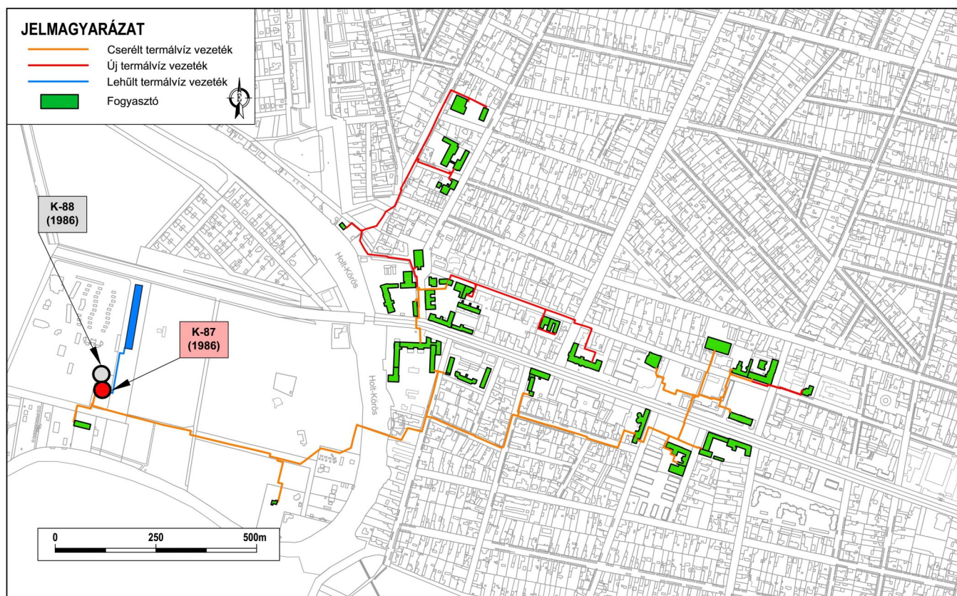
A szarvasi geotermikus rendszer termálkútja, vezetékhalozata és fogyasztói
