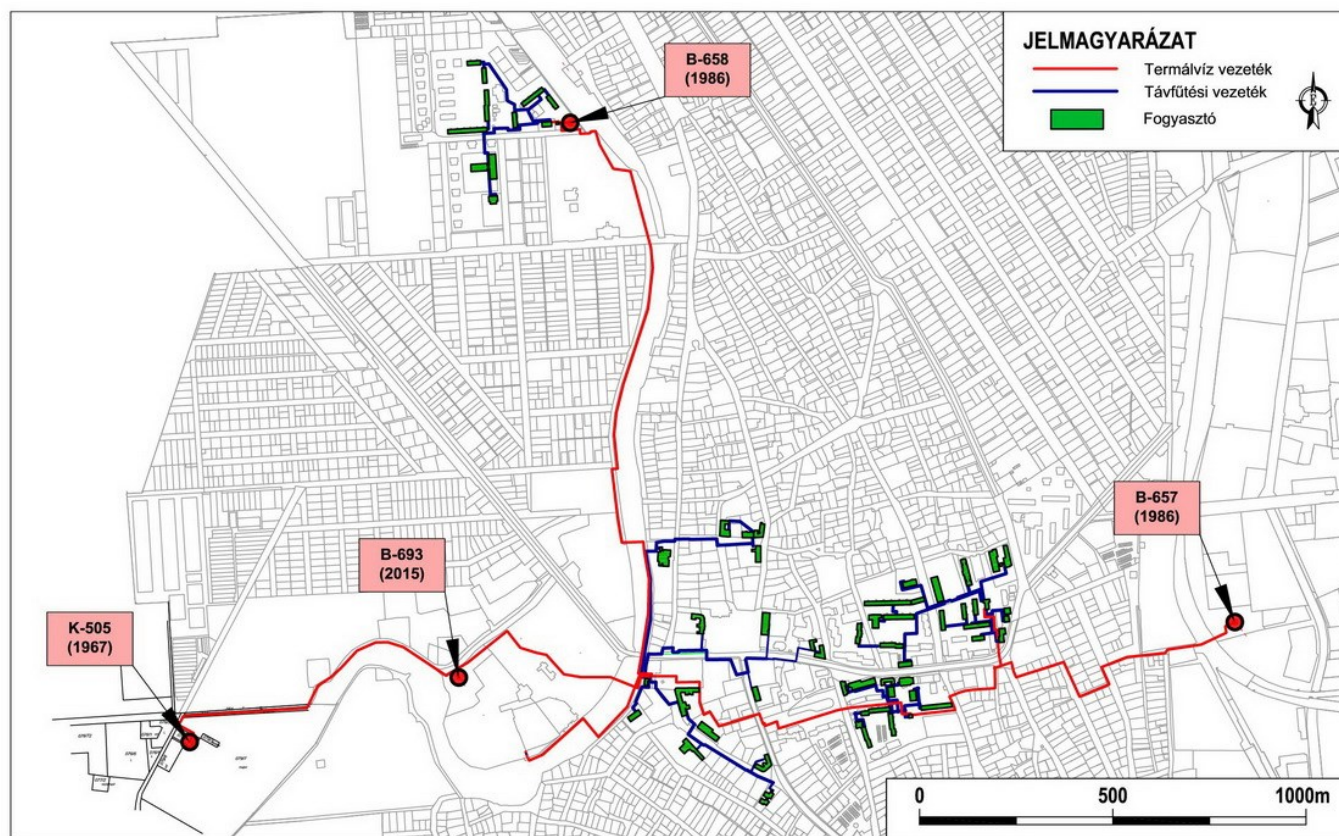
A szentési geotermikus rendszer termálkútjai, vezetékhalózata és fogyasztói
