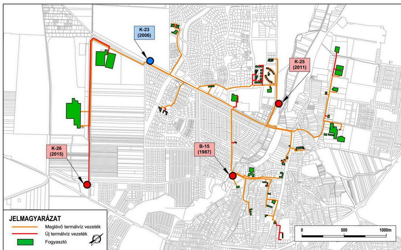
A veregyházi geotermikus rendszer termálkútjai, vezetékhálózata és fogyasztói
