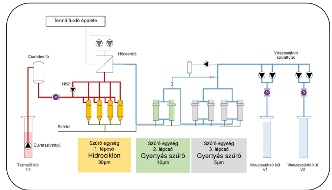
2. ábra Felszíni termál technológia elvi kialakítása Gyopároson
