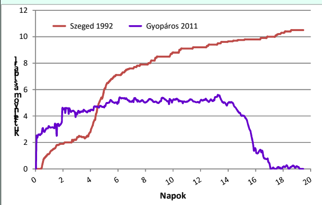
1. ábra A kútfejnyomás alakulása Szegeden és Gyopároson
