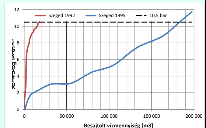
2. ábra A kútfejnyomás alakulása Szegeden 1992-ben és 1995-ben
