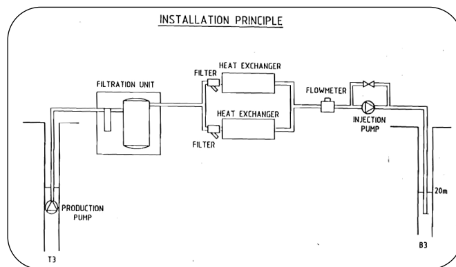
1. ábra Felszíni termál technológia elvi kialakítása
