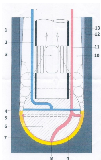
Az olvasztófej függőleges metszete (lépték nélkül)
