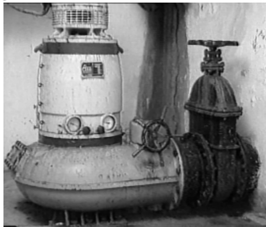
A kísérleti gépcsoport
