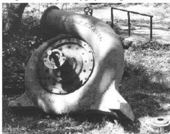
A kibővített Poledniák-féle vízturbina
