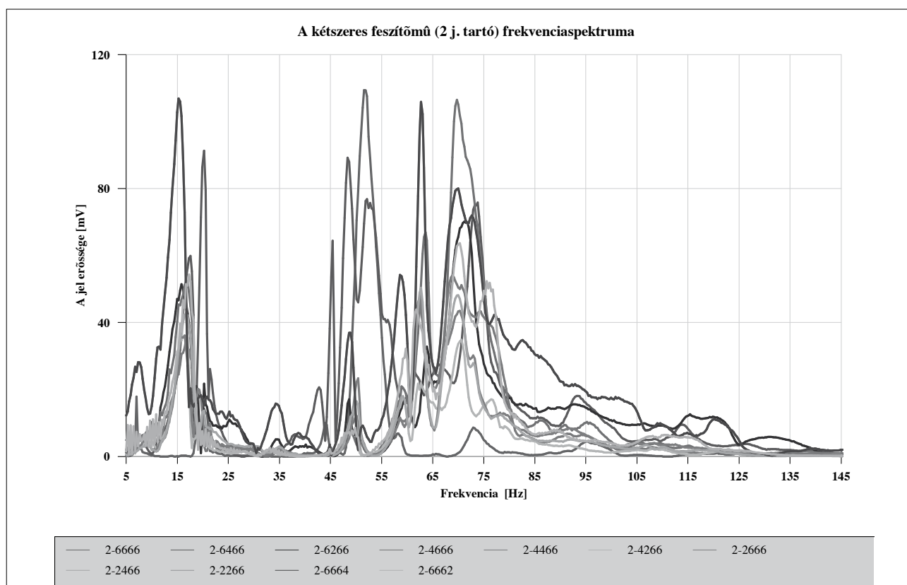
4. ábra A kétszeres feszítőmű frekvenciaspektruma
