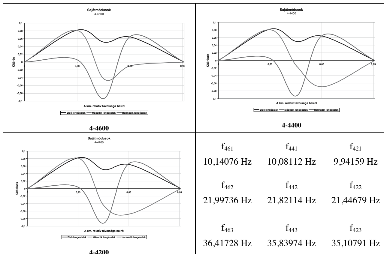
10. ábra A 4-4...j. gerenda sajátmódusai. (A kitérések nagysága mm-ben van megadva.)
