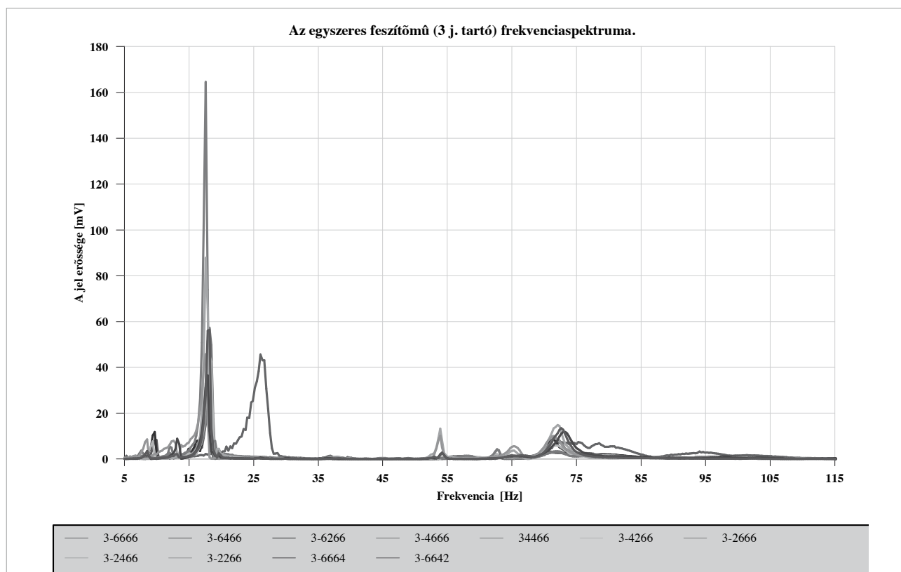
5. ábra Az egyszeres feszítőmű frekvenciaspektruma
