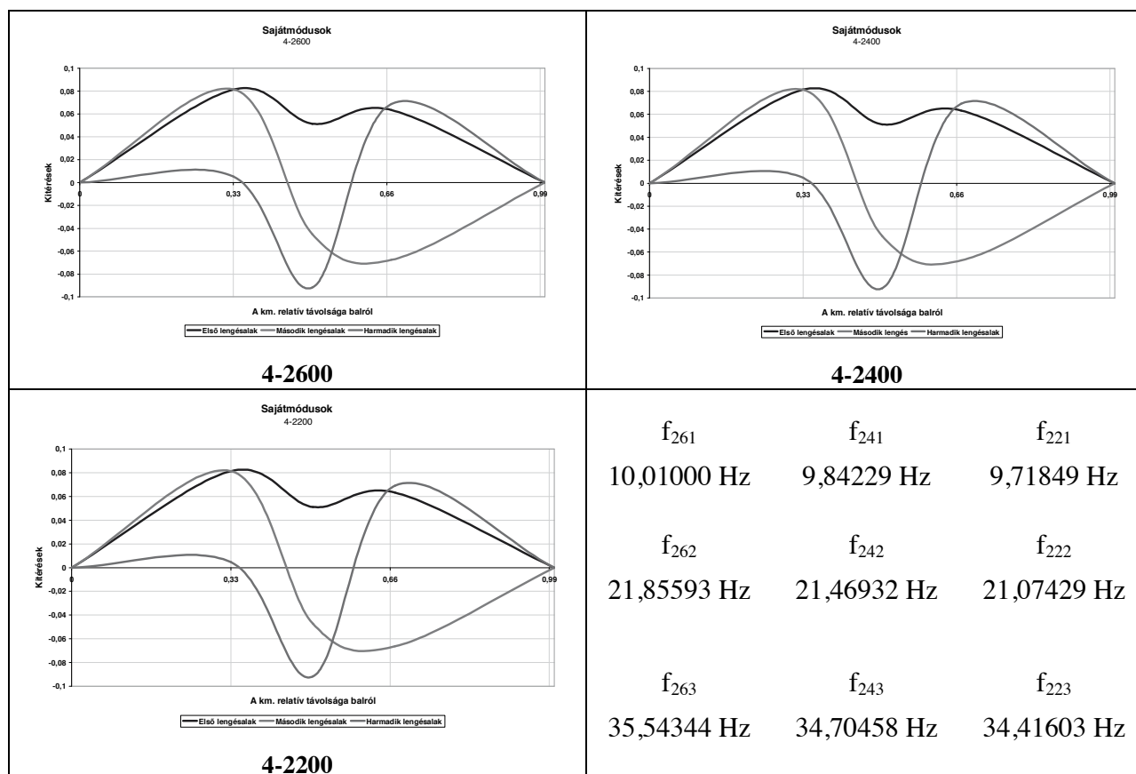
11. ábra A 4-2...j. gerenda sajátmódusai. (A kitérések nagyságát mm-ben adtam meg.)
