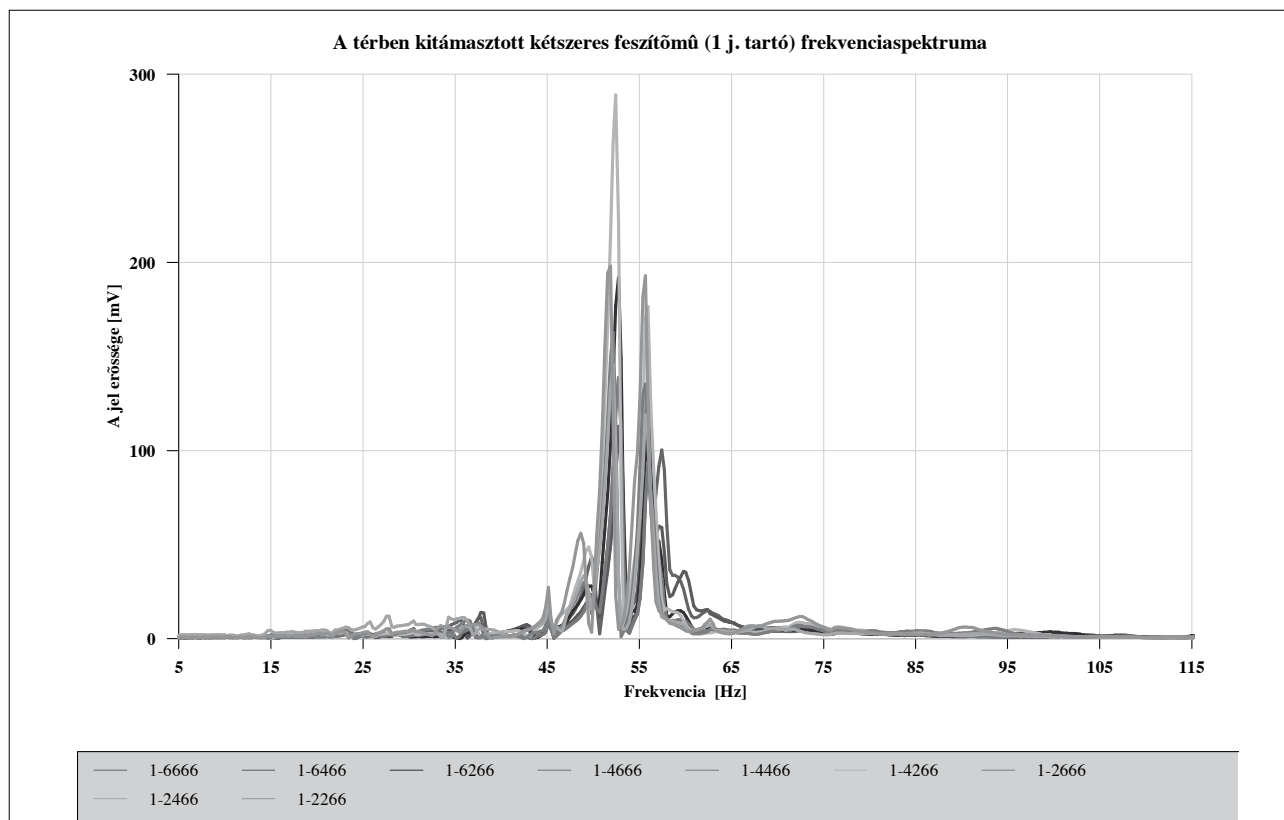
3. ábra A térben is kitámasztott kettős feszítőmű frekvenciaspektruma
