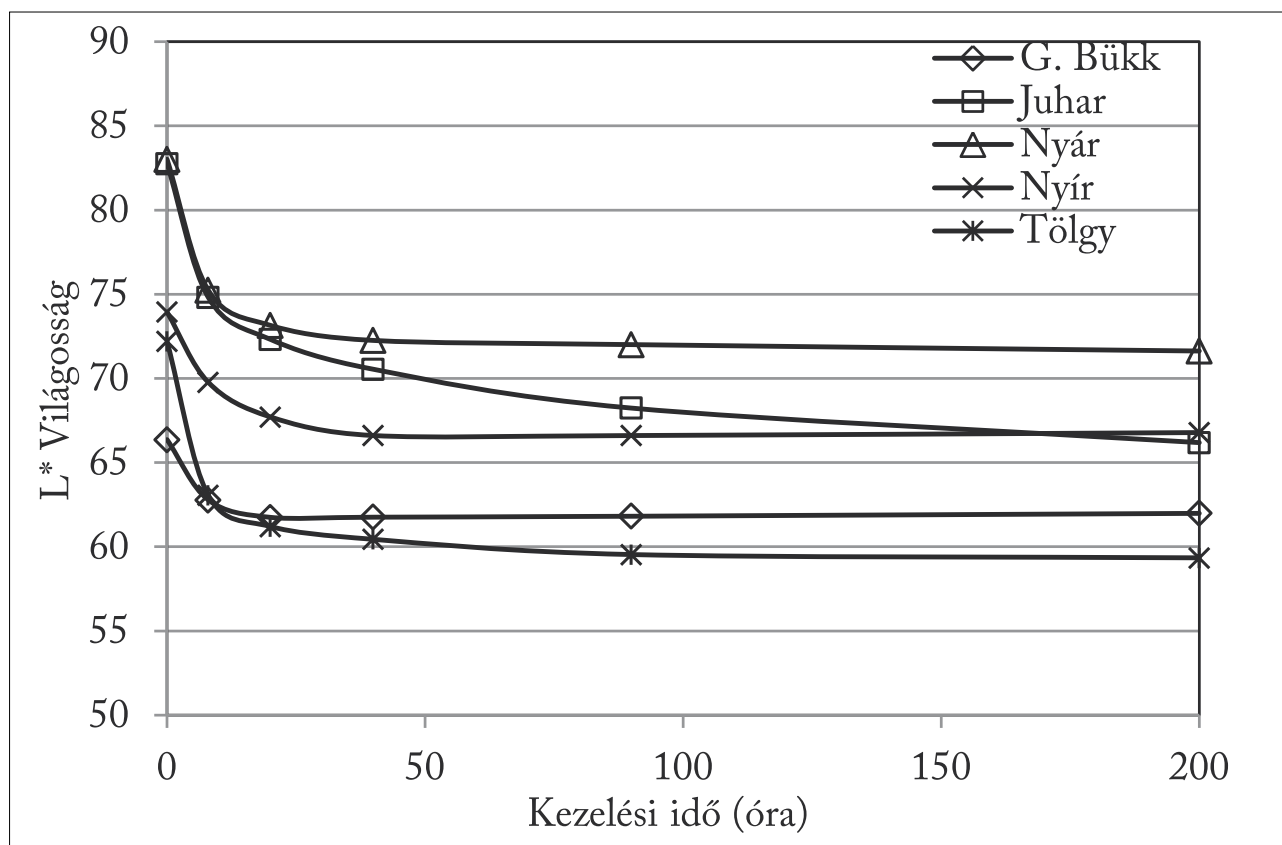
10. ábra A gőzölt bükk, juhar, nyár, nyír és a tölgy világosságának változása higanygőz lámpás besugárzásnál Figure 10 The lightness change of steamed beech, maple, poplar, birch and oak samples caused by mercury lamp irradiation
