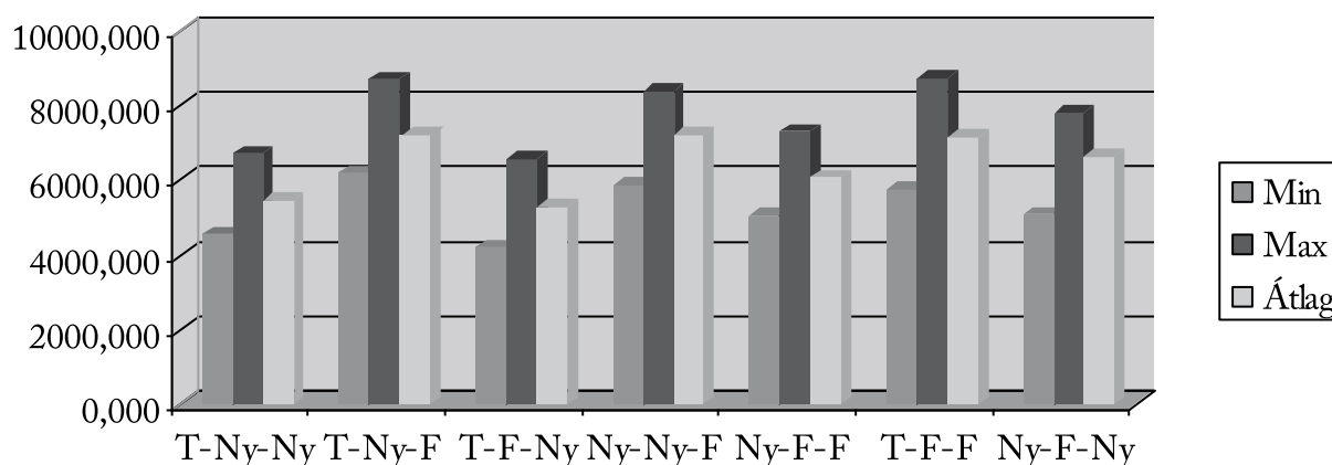
2. ábra A különböző szerkezetű szalagparketták statikus hajlító rugalmassági modulusai
