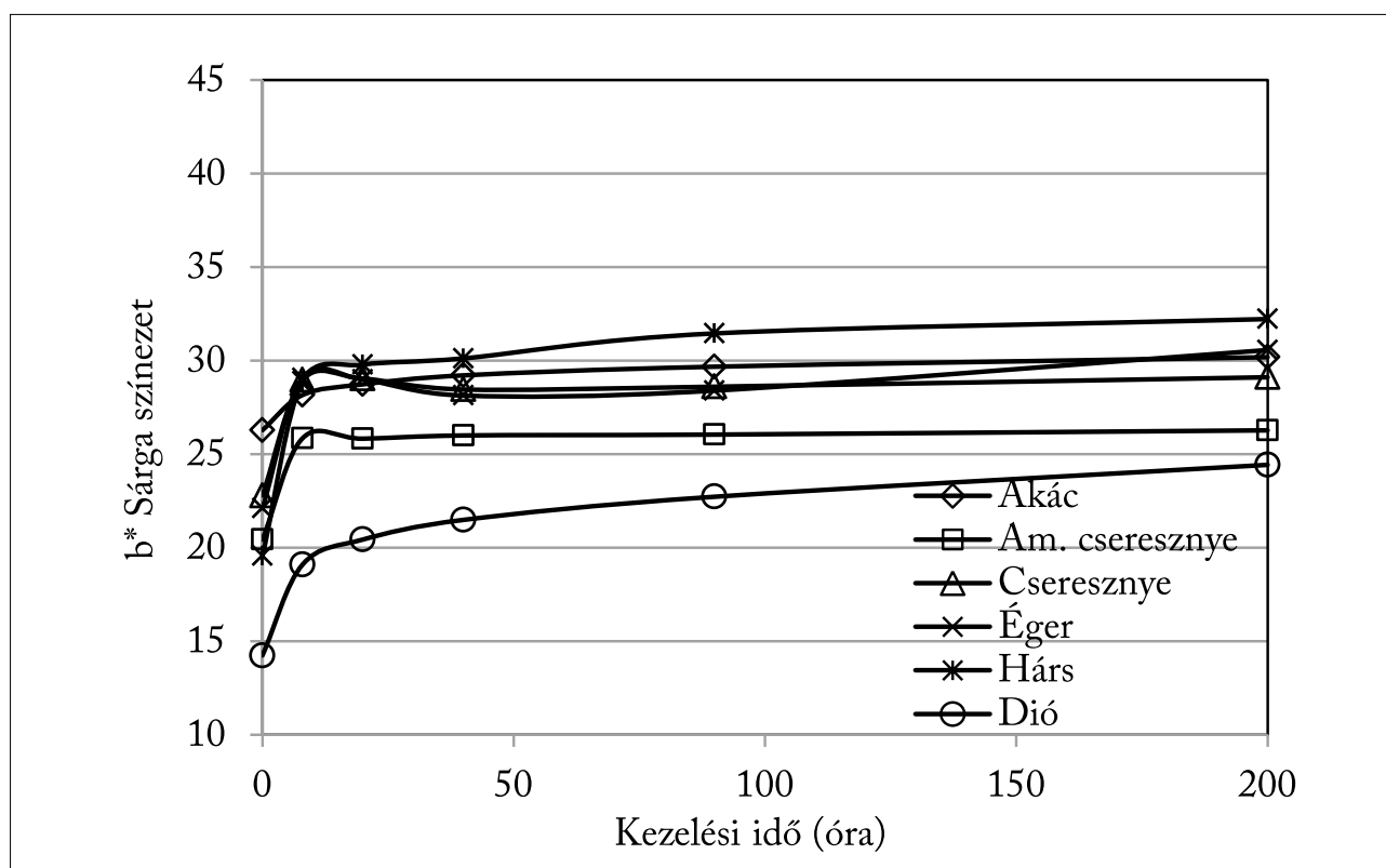
6. ábra Az akác, az amerikai cseresznye, a cseresznye, az éger, a hárs és a dió sárka színezetének változása higanygőz lámpás besugárzásnál Figure 6 The yellowness change of black locust, american cherry, cherry, alder, lime, and walnut samples caused by mercury lamp irradiation
