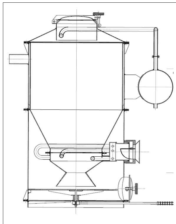
7. ábra Fagásgenerátor terve
