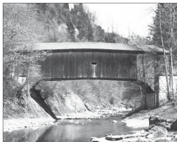
15. ábra A Grubenmann testvérek hídja a Thur mellékágán, ép. 1780. St. Gallen kanton, Svájc (Source: Philip Caston, 2009)
