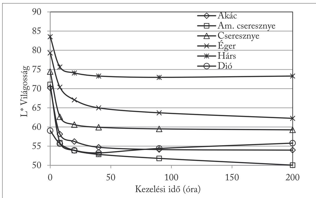
9. ábra Az akác, az amerikai cseresznye, a cseresznye, az éger, a hárs és a dió világosságának változása higanygőz lámpás besugárzásnál Figure 9 The lightness change of black locust, american cherry, cherry, alder, lime, and walnut samples caused by mercury lamp irradiation
