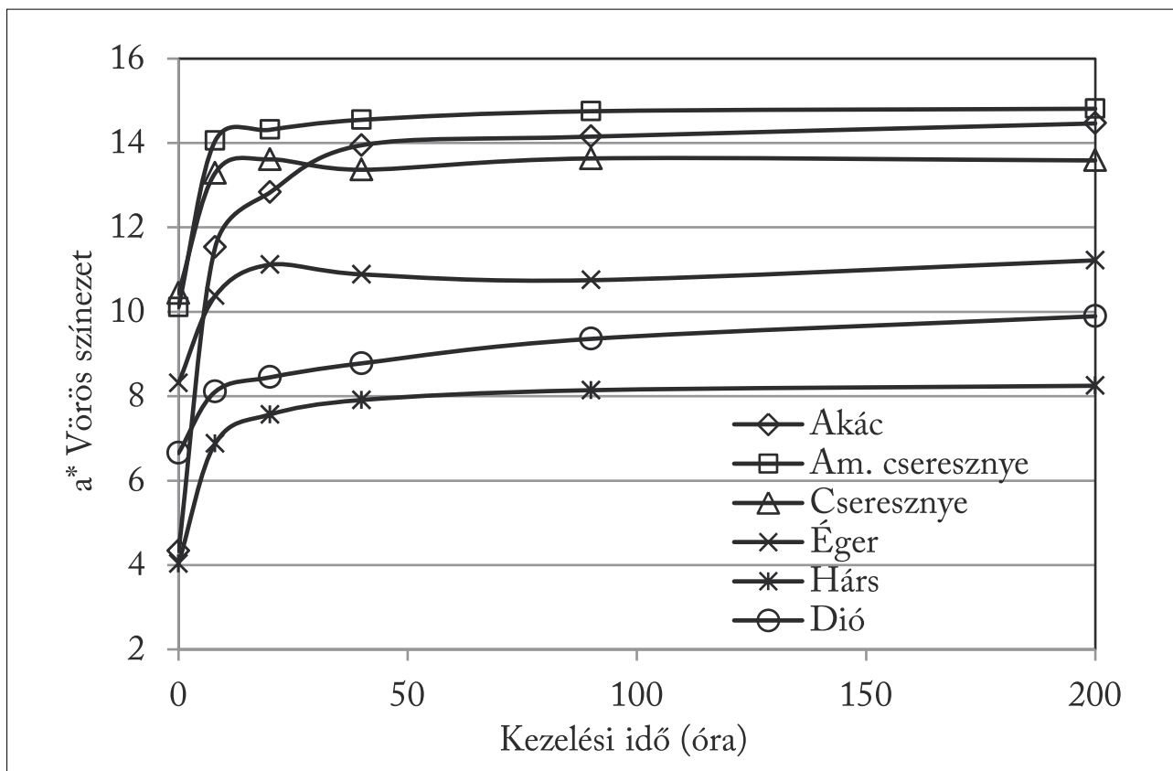
2. ábra Az akác, az amerikai cseresznye, a cseresznye, az éger, a hárs és a dió vörös színezetének változása higanygőz lámpás besugárzásnál
