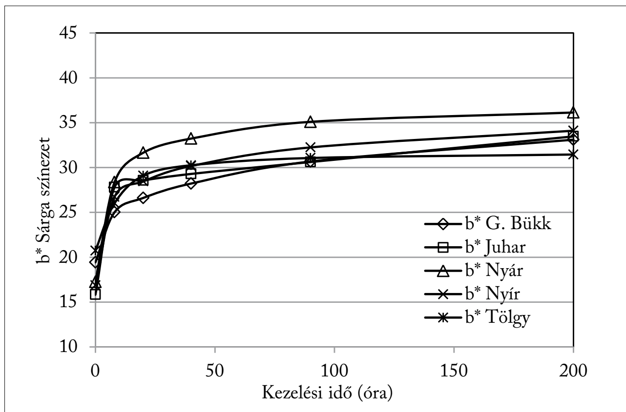
7. ábra A gőzölt bükk, juhar, nyár, nyír és a tölgy sárka színezetének változása higanygőz lámpás besugárzásnál Figure 7 The yellowness change of steamed beech, maple, poplar, birch and oak samples caused by mercury lamp irradiation
