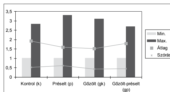
1. ábra Különböző nyár anyagok zsugorodási anizotrópiája Figure 1 Anisotropic shrinkage of different poplar species
