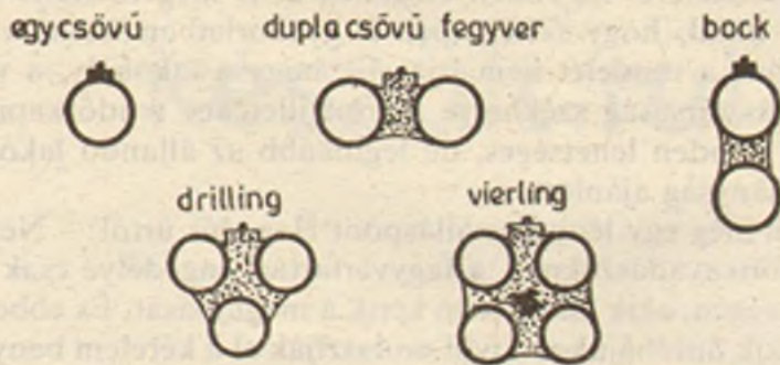
1. sz. ábra. Sörétes fegyvercső-elrendezések
