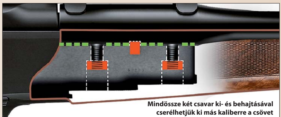
Egyetlen spirálrugó mozgatja az R8-as zárszerkezetét
