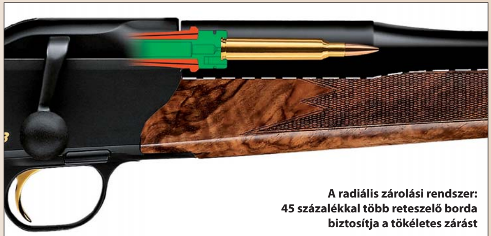
Az egyenes vonalú zárdugattyú lehetővé teszi a gyors ismétlést
