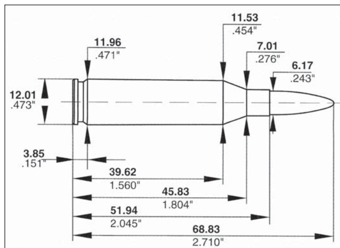
.243 Winchester – méretek milliméterben és inchben
