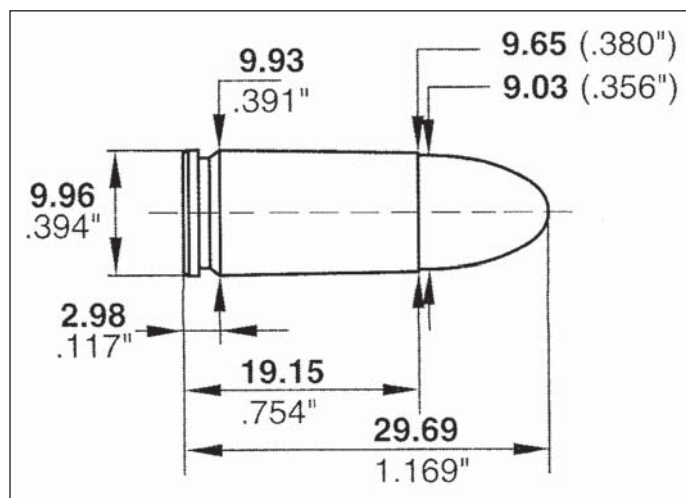
9mm Luger Parabellum – méretek milliméterben és inchben
