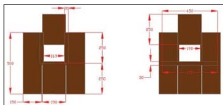
Tető felül- és alulnézet
