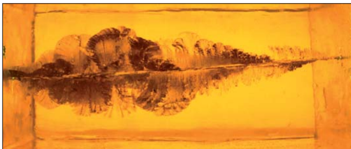
A GECO PLUS (balra) és EXPRESS (jobbra) hatása a ballisztikai zselatin tömbre. Jól látható a mélységi hatás különbözősége
