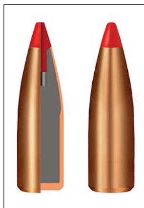
A GECO EXPRESS metszete
