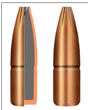
A GECO PLUS metszete
