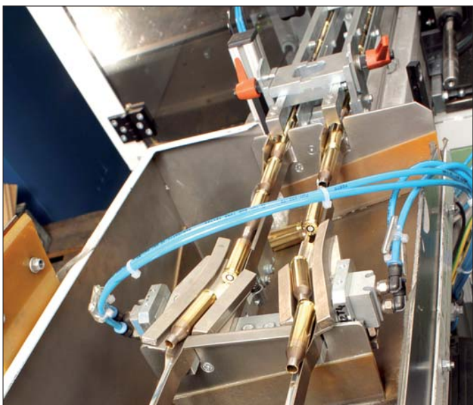
A töltényhüvelyek adagolása a töltőautomatába
