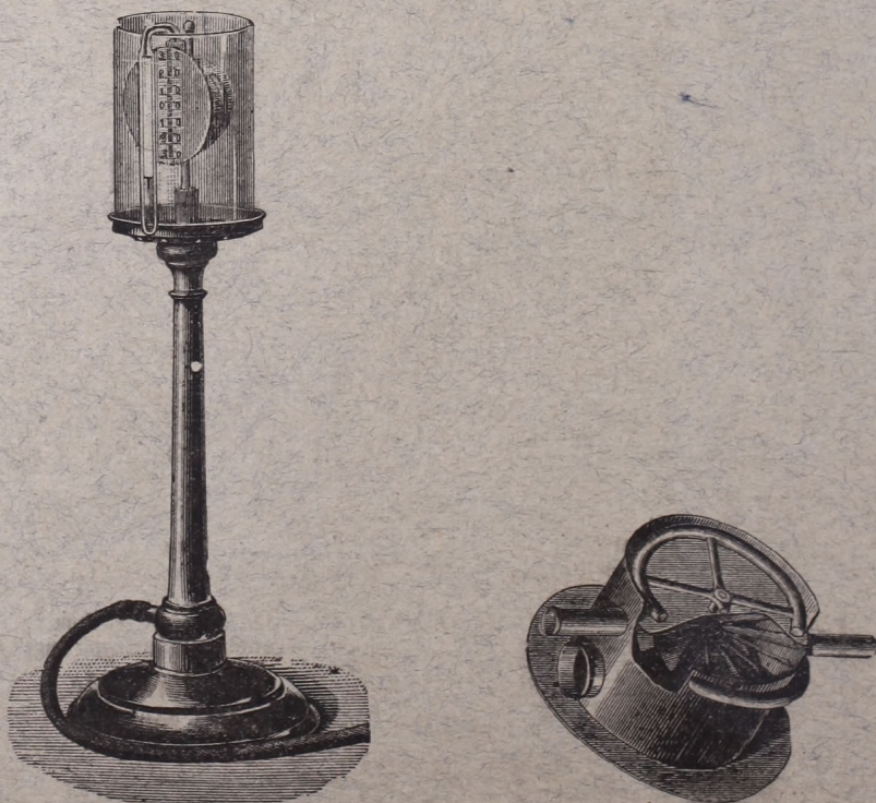
A Lambrecht-féle harmatpont-tükör.
