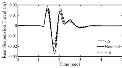
(a) AVSS
