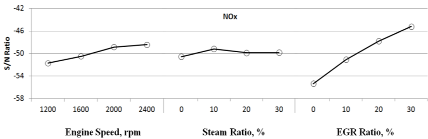
Figure 2 (d) S/N values of factor levels for NOx
