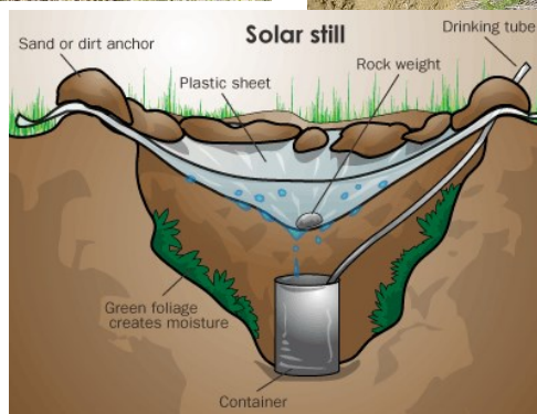
57. kép: Vízszerezés párologtatással. 17
