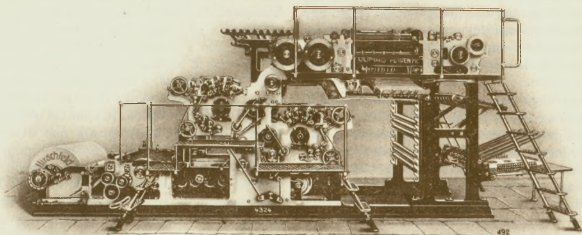
A Vogtländische Maschinenfabrik AG., Plauen i/V, egy tekercsről elő- és hátnyomást egy menetben végző, egy színt nyomtató offsetkörforgógépe, hajtogató- és ívkirakószerkezettel — Einrollen-Offsetrotationsmaschine der Vogtländischen Maschinenfabrik AG., Plauen, für gleichzeitigen einfarbigen Schön- und Widerdruck mit Falzapparat und Planoauslage
