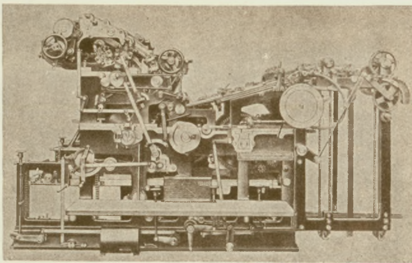
1—2. ábra. Schnellpressenfabrik Frankenthal Albert Cie AG., Frankenthal, gépgyár egyszerű egyszerű nyomó egyszerű offsetkörforgógépe — Abb. 1—2. Einfache Offsetrotationsmaschine für einfurbigen Druck der Schnellpressenfabrik Frankenthal Albert & Cie AG., Frankenthal
