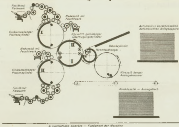
A nyomtatógép alapváza — Fundament der Maschine
