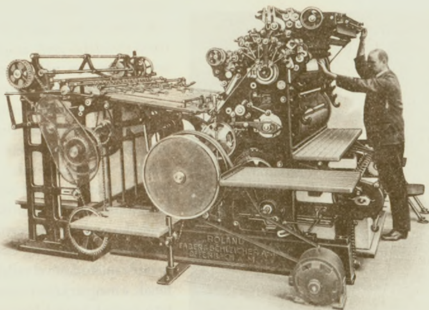
A Faber & Schleicher AG., Offenbach a/M., gépgyár »Rolanda« offsetnyomógépe — Gummidruckpresse »Rolanda« der Druckmaschinenfabrik Faber & Schleicher AG., Offenbach a/M.
