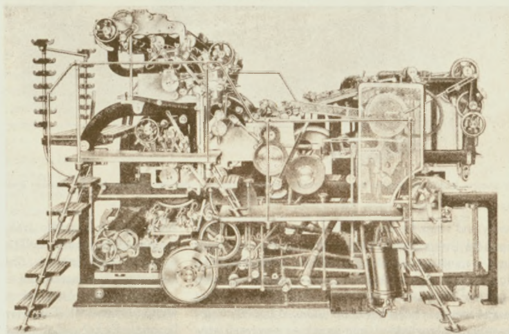
5—6. ábra. A Schnellpressenfabrik Frankenthal Albert & Cie AG., Frankenthal, cég készítő elő- és hátnyomást egyszerre végző offsetkőforgógépe — Abb. 5—6. Offsetrotationsmaschine für gleichzeitigen zweifarbigen Schön- und Widerdruck der Schnellpressenfabrik Frankenthal, Albert & Cie AG., Frankenthal
