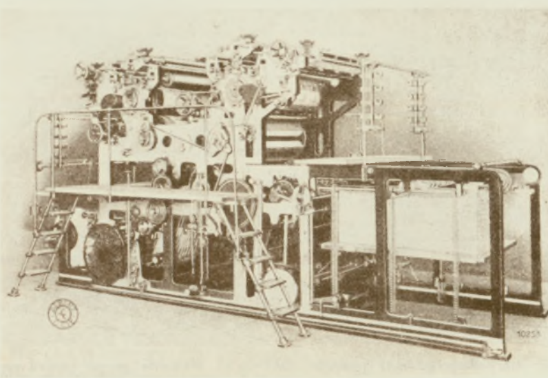
3. ábra. A Schnellpressenfabrik Frankenthal Albert Cie AG., Frankenthal, gépgyár egy tekercspapírosra két színt nyomó, változtatható alakú offsetkőforgógépe — Abb. 3. Variabel-Einrollen-Offsetrolationsmaschine für Zweifarbendruck der Schnellpressenfabrik Frankenthal Albert & Cie AG.
