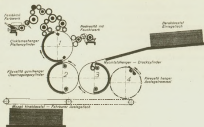
A nyomtatógép alapváza — Fundament der Maschine
