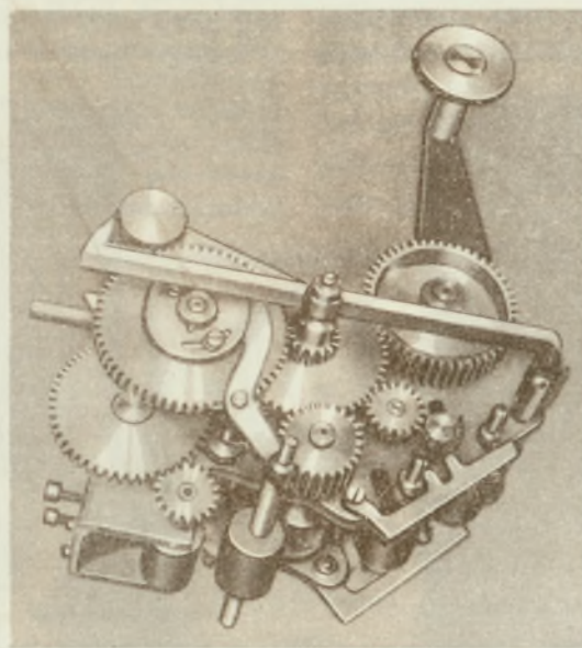
A »Typar« írószedőgép festékezőszerkezete — Farbwerk der »Typar« Schreibsetzmaschine
