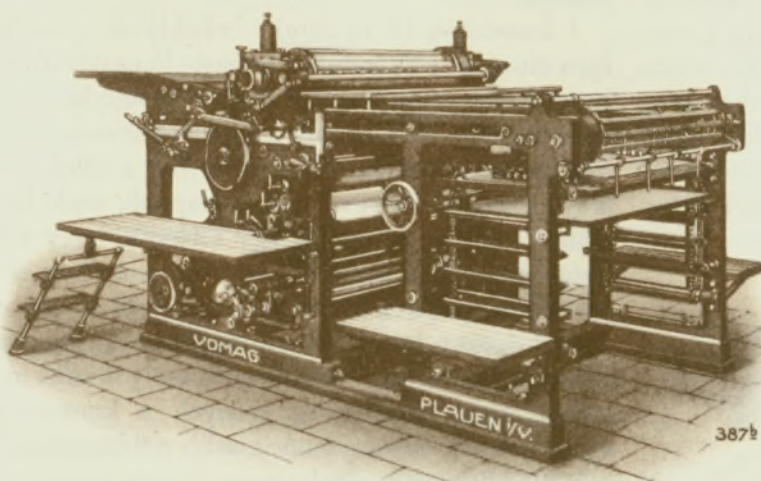
A Vogtländische Maschinenfabrik AG., Plauen i/V., gépgyár »Vogtland« nevezetű kéthengeres offsetnyomógépe tüberakásra — Zweizylinder-Offsetmaschine für Bogenanlage »Vogtland« der Vogtländischen Maschinenfabrik AG., Plauen i/V.
