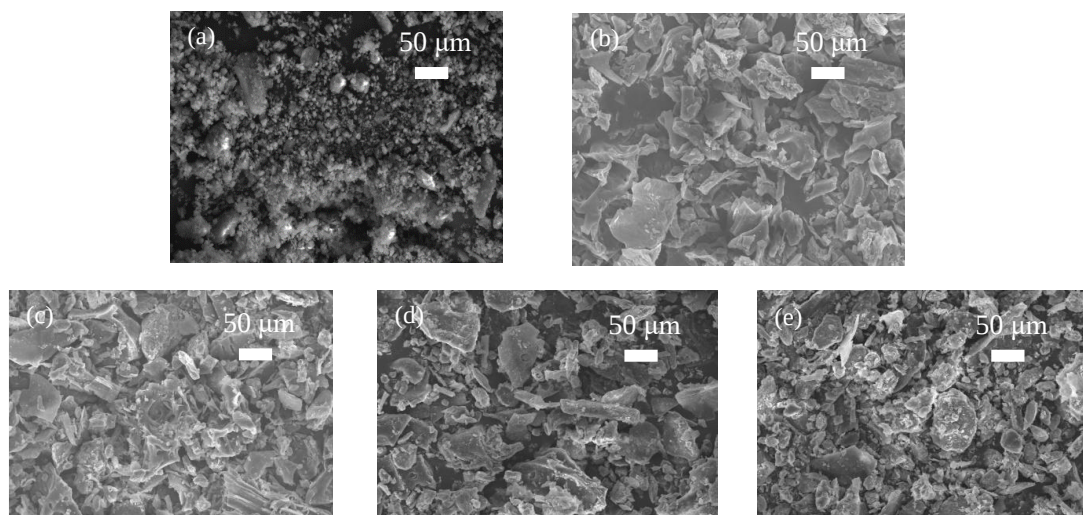
Figure 4. SEM images of (a) PAL, (b) BC, (c) BP21, (d) BP11, (e) BP12
