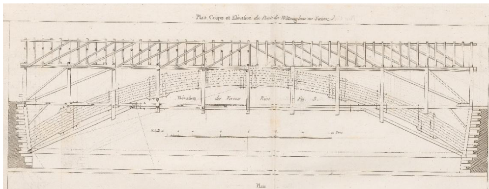
6. kép. Grubenmann 1764-ben ácsolt wetztingeni ívhídja a Limmat folyón. 12
