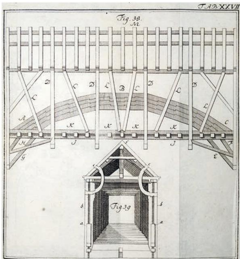
5. kép. Silberschlag rajza egy tömör gerendaívról. 10
