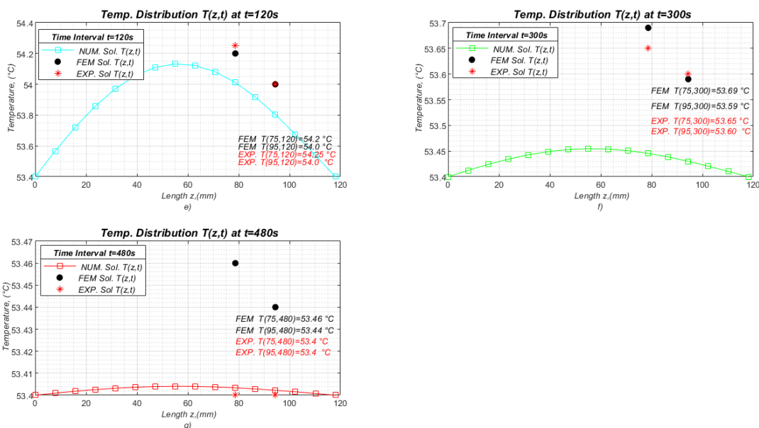
Figure 9. Transient state analysis e) \Delta t = 120\text{ s} , f) \Delta t = 300\text{ s} , g) \Delta t = 480\text{ s} .
