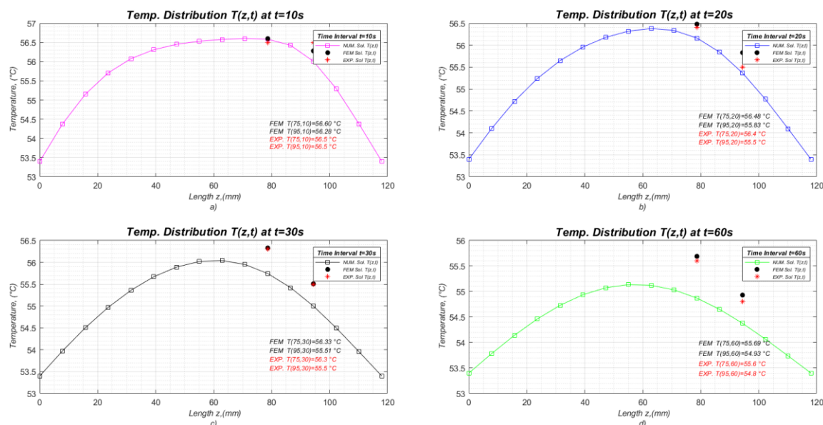
Figure 8. Transient state analysis a) \Delta t = 10\text{ s} , b) \Delta t = 20\text{ s} , c) \Delta t = 30\text{ s} , d) \Delta t = 60\text{ s} .
