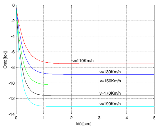
4.9 ábra A orsózó szögsebesség átmeneti függvénye
