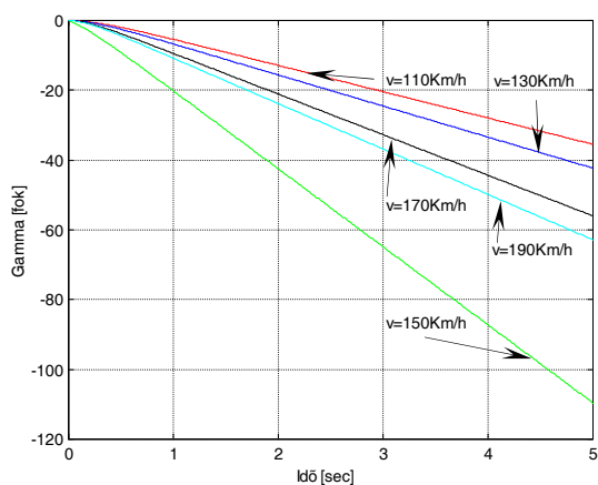
4.10 ábra A bedöntési szög átmeneti függvénye
