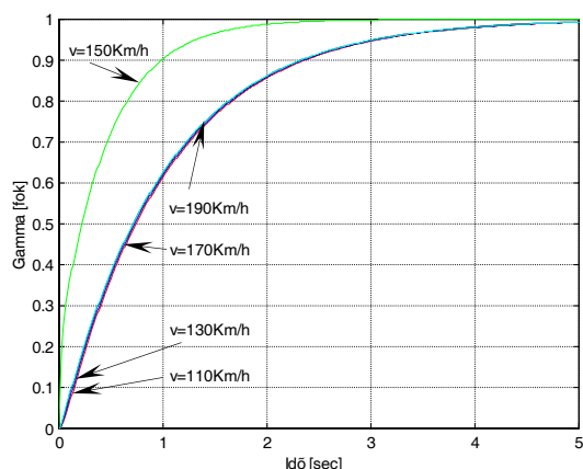
5.5 ábra A bedöntési szög átmeneti függvénye
