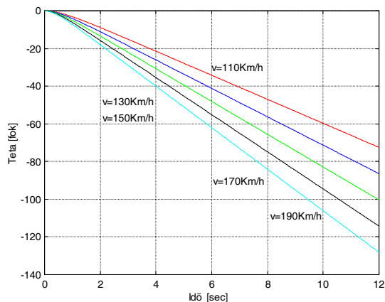
4.6 ábra A bólintási szög átmeneti függvénye
