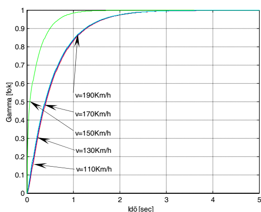
5.7 ábra A bedöntési szög átmeneti függvénye
