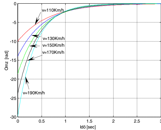
4.2 ábra A bólintási szögsebesség impulzusválasz függvénye
