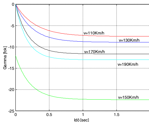
4.5 ábra A bedöntési szög impulzusválasz függvénye
