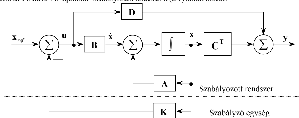
2.1 ábra A teljes állapot—visszacsatolású szabályozási rendszer hatásvázlata
