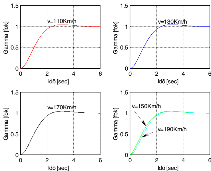
6.2 ábra A bedöntési szög átmeneti függvényei
