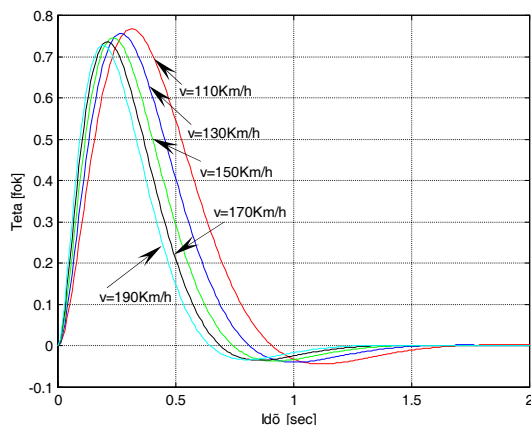
5.1 ábra A bólintási szög átmeneti függvénye
