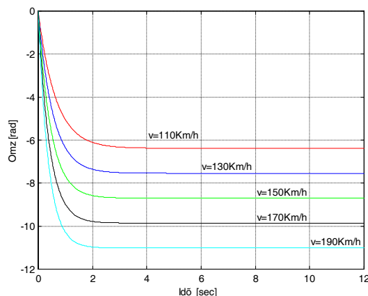
4.7 ábra A bólintási szögsebesség átmeneti függvénye
