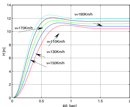
5.3 ábra A magasság átmeneti függvénye
