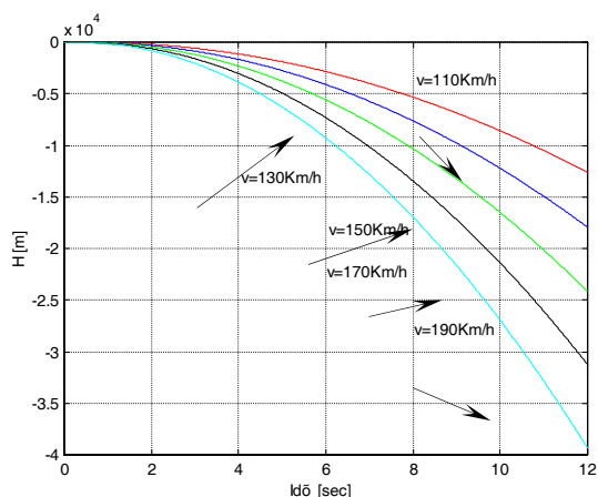
4.8 ábra A magasság átmeneti függvénye
