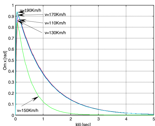
5.4 ábra Az orsózó szögsebesség átmeneti függvénye
