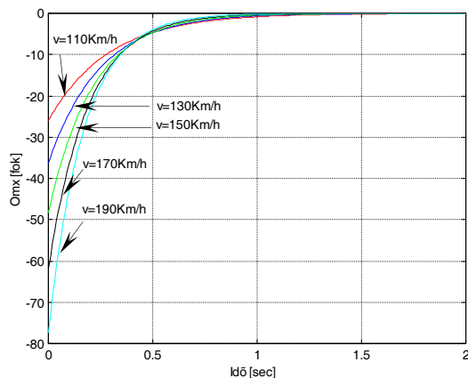
4.4 ábra A orsózó szögsebesség impulzusválasz függvénye
