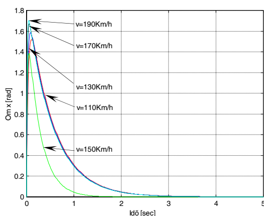
5.6 ábra Az orsózó szögsebesség átmeneti függvénye
