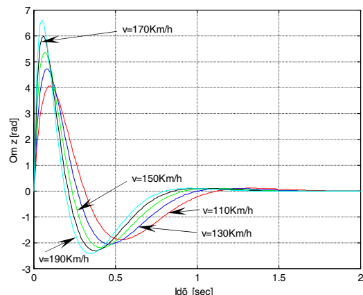
5.2 ábra A bólintási szögsebesség átmeneti függvénye
