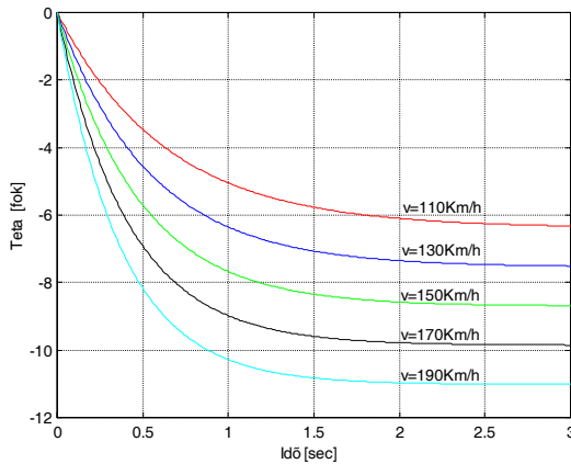
4.1 ábra A bólintási szög impulzusválasz függvénye
