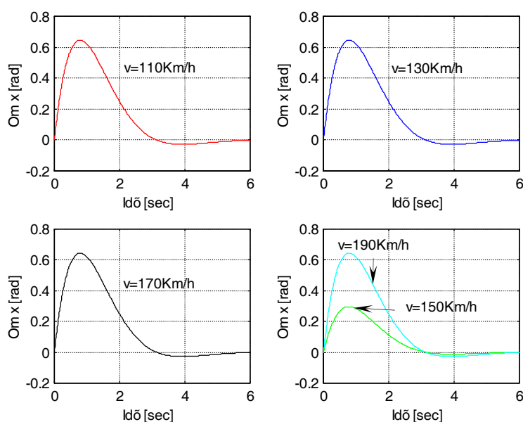
6.1 ábra Az orsózó szögsebesség átmeneti függvényei
