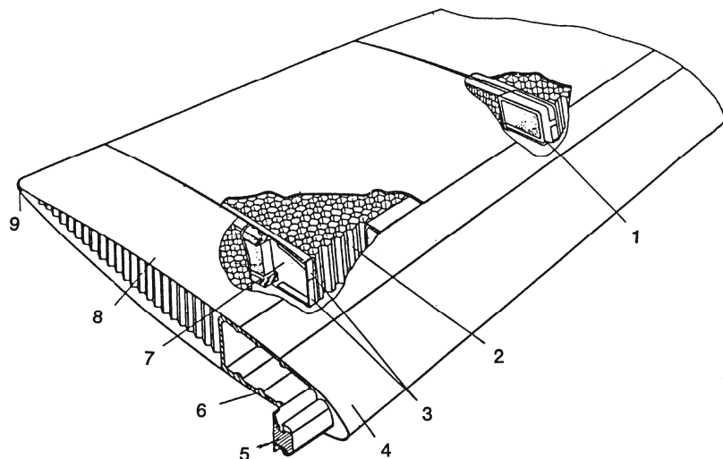
6. ábra. Helikopter forgószárnylapát felépítése: 1. Rekeszközi betét, 2. Sejtrácsos töltőanyag, 3. Talp, 4. Jégtelenítő, 5. Ellensúly, 6. Főtartó, 7. Borda, 8. Borítás és 9. Hátsó hosszmerevítő
