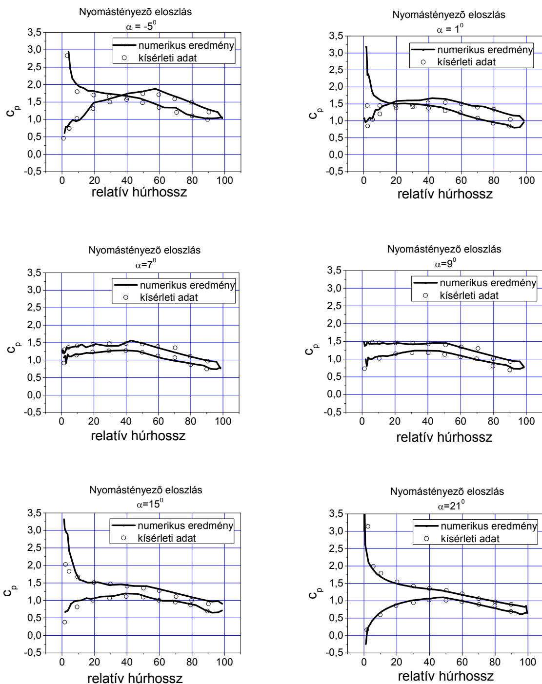
6. ábra. Nyomás tényező a relatív húrhossz függvényében különböző állásszögek esetén ( \beta_l=30^\circ and Re=2,45e5 , v_{inf, inlet}=29 m/s, folytonos vonal: számítás eredménye, körök: mérés [4])
