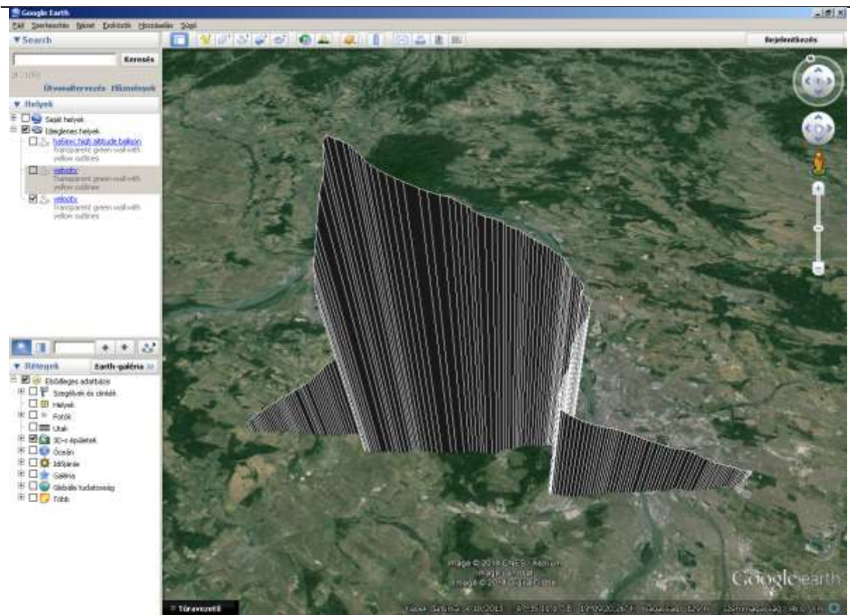
A maximális magasság 30724 méter, ahol a ballon kidurrant és a mérőrendszer elkezdett viszázuhanu a Földre.
