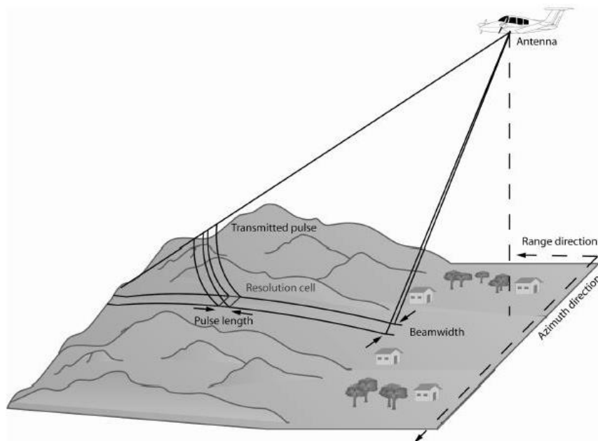
10. ábra Képképzés a repülőgépre szerelt SAR rendszereknél 21
