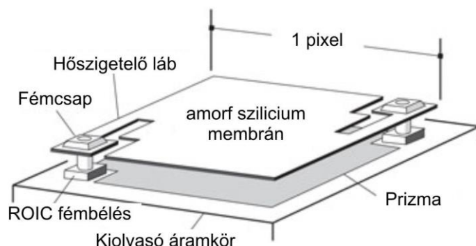
9. ábra Amorf szilícium elemi mikrobolométer érzékelő felépítése 20
