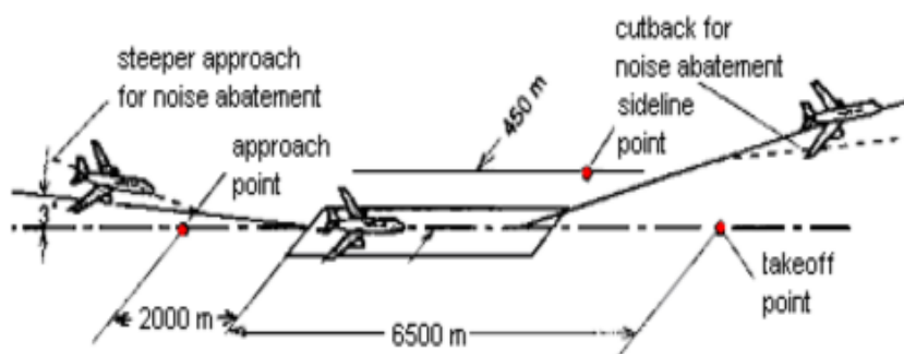
8. ábra Légijárművek zajmérőpontja a zajminősítés során
