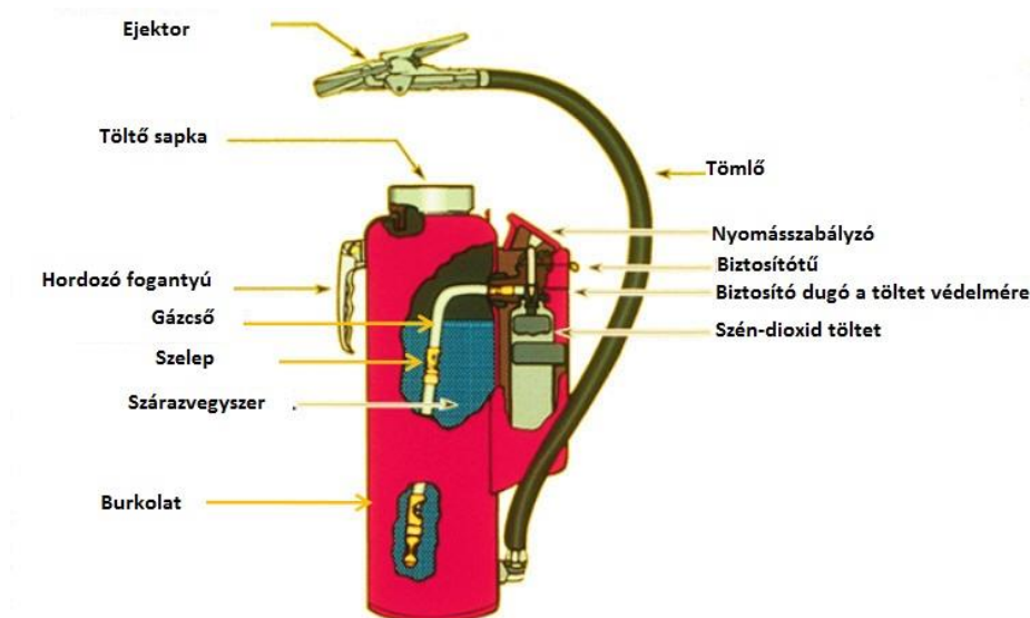
2. ábra Kézi porraloltó készülék robbantott ábrája 6 [7]
