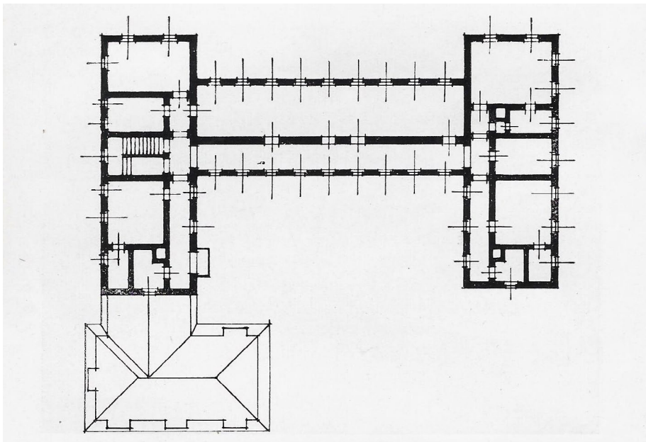
4. kép – A klinika vázlatos alaprajza az utóbb készített pótépületszárnyal
