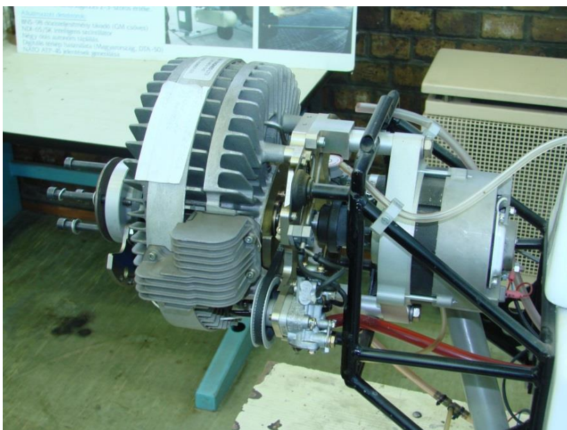
10. számú ábra. A Szojka Wankel-motorja önálló olajkenési rendszerrel rendelkezik
