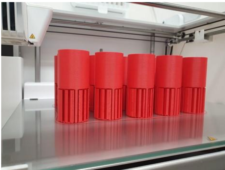
4. számú ábra. Kumulatív töltetházak 3D nyomtatása. Forrás: a szerzők felvétele
