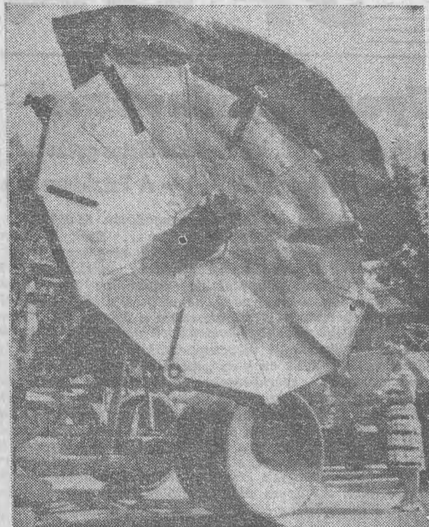
„DMK-3-nak hívják ezt az érdekes, tárcsás gépet, melyet tőzegkitermelésre szerkesztettek. Traktorvontatással 7 óra alatt két kilométer hosszú, 120 centiméter mély árkot tud kiásni
