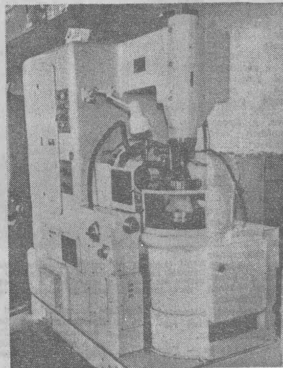
Felautomata fogazógép. A vityebszki gépgyár készítménye, egyenes és ferdefogazású homlokkerekek megmunkálására. A gép gyorsított számmozgatással dolgozik, és a marót tengelyirányban automatikusan átállító készülék is van rajta
