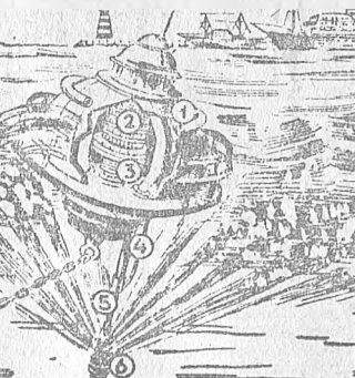
Az önműködő légsűrítési bóják szerkezete: 1. bója, 2. kompresszorhenger, 3. sűrítődugattyú, 4. hajlékony légvezeték, 5. főnyomócső, 6. szelepek, 7. ellátott hullámtörő, 8. horgonyléc, 9. horgony.
