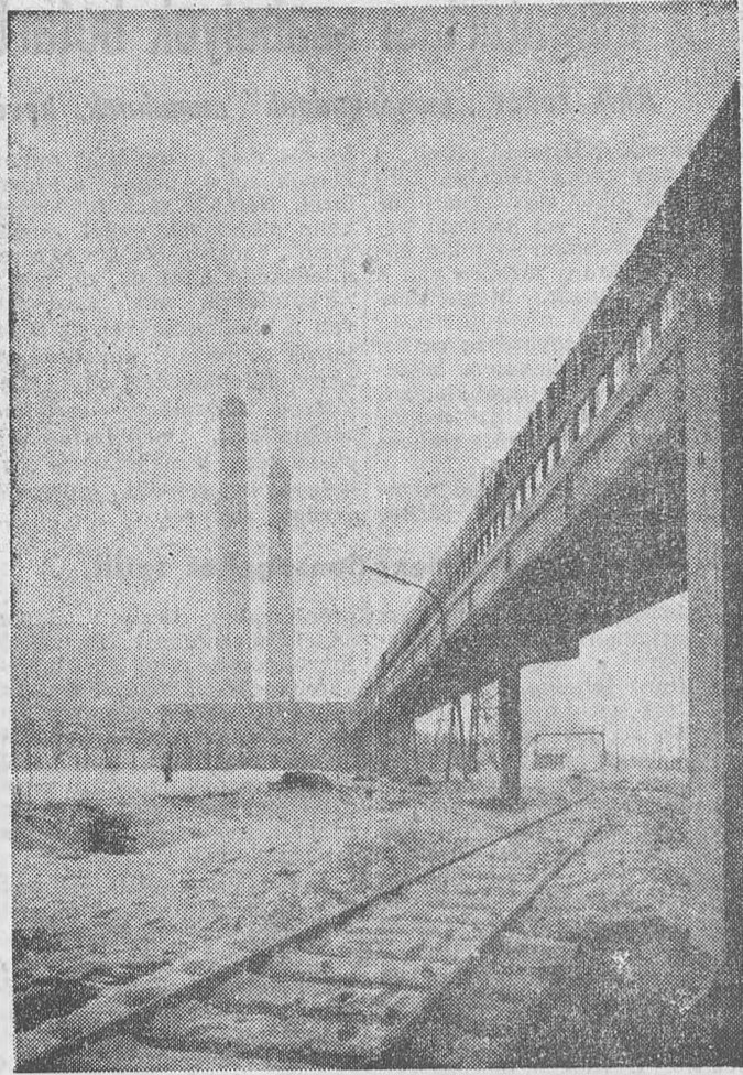
Decemberben adták át rendeltetésének az Ajkai Hőerőművet. Bővítésére, amelyet még 1956-ban kezdtek meg, több mint egymillió forintot fordítottak. A hőerőmű teljesítménye most a bővítés előtt 57 megawattal szemben 150 megawatt. Teljes berendezése, a mesterséges szellőzésű hűtőtornyokkal együtt magyar gyártmány.
