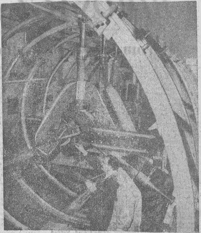
Új bányagép mintapéldánya készült el, a szénbányászat „rakétája”. Az új gép meggyorsítja a vágathajtást és nyomában azonnal beépíthető a biztosítószerkezetek. Kipróbálására egy bányafolyosó utánzatot építettek meg, amelyben a gép mozoghat.
