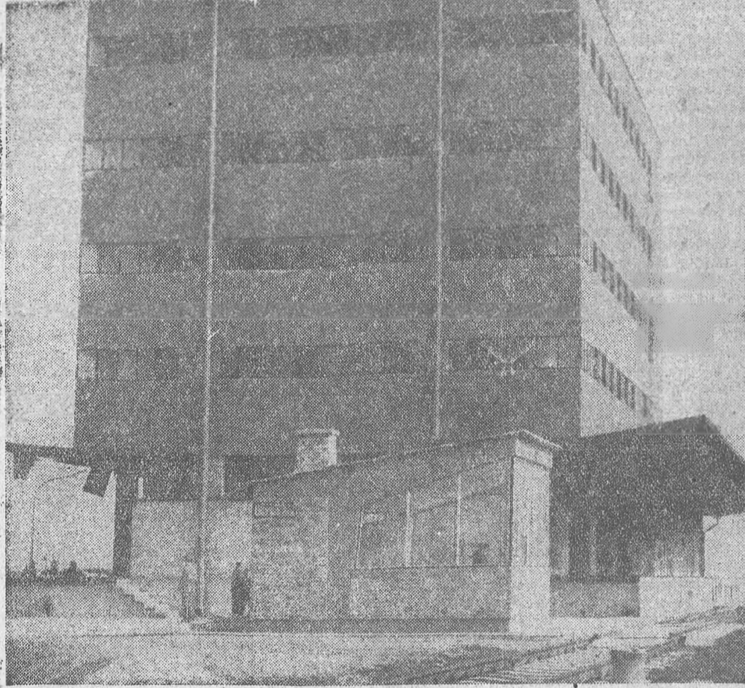
A Szolnok megyei Ujszászon, a vasútállomás közvetlen közelében a kitűzött kétéves határidő alatt felépítették az ország ez idő szerint legkorszerűbb gabonatarolóját. A 23 milliós beruháással elkészült hatalmas épület harminc méter magasba szökkenő 18 szilójában és az emeletek földemjén nem kevesebb, mint hatszáz vagon szemesterményt lehet tárolni. Ujszász és környéke, az egész járás ideszállíthatja majd a termést, a vasútállomásra érkező szerelvényeket külön iparvágányon tolathatják a tárházhoz. A tárházban minden mozgatóeszköz géppel végző, központi vezérlő terem asztaláról egybenyomással irányítják a munkát.
