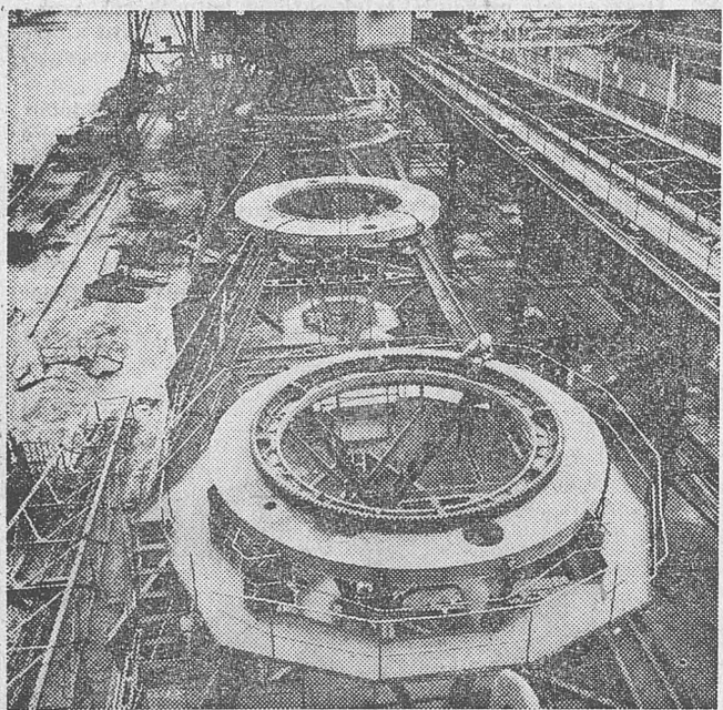
A Magyar Hajó- és Darugár darugáregységében sorozatban készítik exportra az 5 tonna teherbírású, 30 méter gémkinyúlású darukat. Az idén hatvanat gyártanak szovjet megrendelésre. Képünkön: sorozatban készülnek az exportdaruk.
