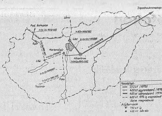
750/400 kV-os energiaátvitellel kapcsolatos hálózati létesítmények
