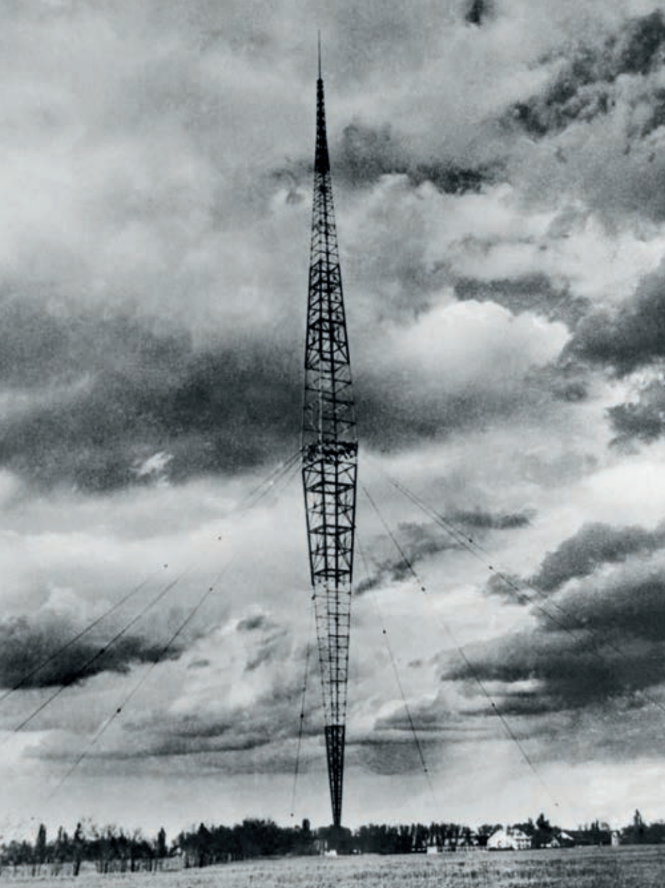
Lakihegyi rádióállomás, a 314 m magas Blow-Knox rendszerű antenna. Forrás: postamuseum.hu
