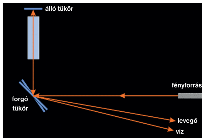
A fénysebesség-különbség kimutatására szolgáló, forgó tükrös módszer vázlata (physics.stackexchange.com)
