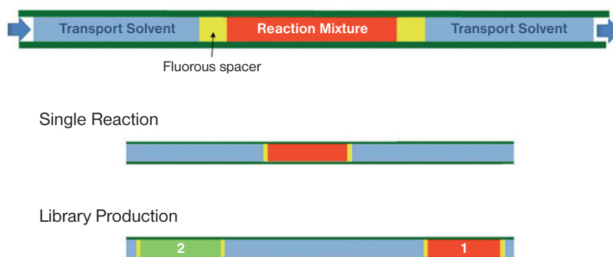
7. ábra. A fluoros oldószerrel szétválasztott folyadékarambok (cseppek) lehetőséget nyújtanak gyors egymást követő reakcióra és könyvtárszintézisre
