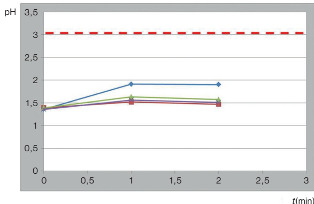
5. ábra. Gyári lúgosító kapszula hatékonyságának vizsgálata (kék: 0,5 g \text{CaHPO}_4 \cdot 2\text{H}_2\text{O} ; zöld: ~0,6 g kapszula-töltőanyag; lilá: 0,5 g kapszula-töltőanyag; piros: ~0,3 g kapszula-töltőanyag)
