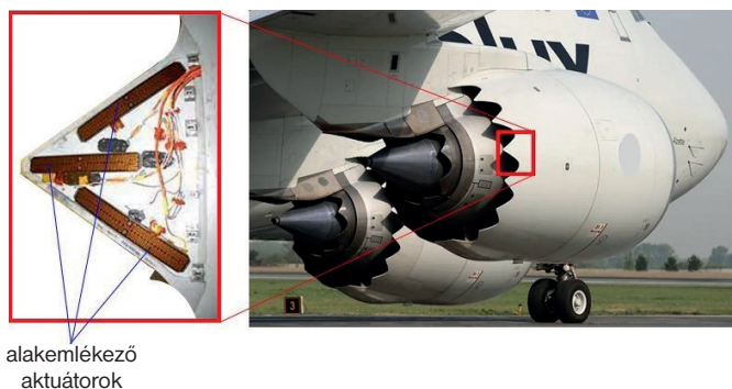
5. ábra. Változó geometriájú borítódíom – részben belülről – a sugárhajtómű hátsó részén
