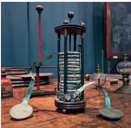
6. ábra. A Volta-oszlop (cink- és ezüst-korongok sora egymásra rakva, egy-egy cink-ezüst párost sóoldattal átitatott filc vagy kartonpapír választ el)
