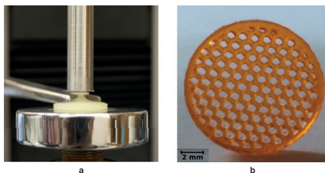
4. ábra. Nyálkahártya-analóg hidrogél mukoadhéziós kísérletekhez (a) és enzimrögzítésre használható pórusos vázszerkezet (b)
