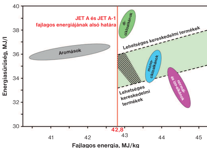
4. ábra. Szénhidrogéncsoportok/elegeik energiasűrűsége és fajlagos energiája (az ábra saját módosítás és szerkesztés [8] alapján)
