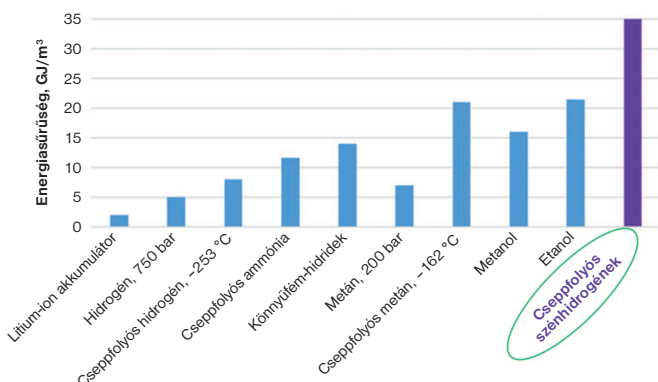
3. ábra. Különböző motorhajtóanyagok energiasűrűsége [7]
